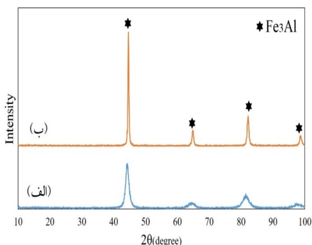
شکل 2- الگوهای XRD سیستم دوتایی Fe-Al بعد از الف - 30 ساعت آسیاب‌کاری و ب- پس از انجام عملیات روکش‌کاری
