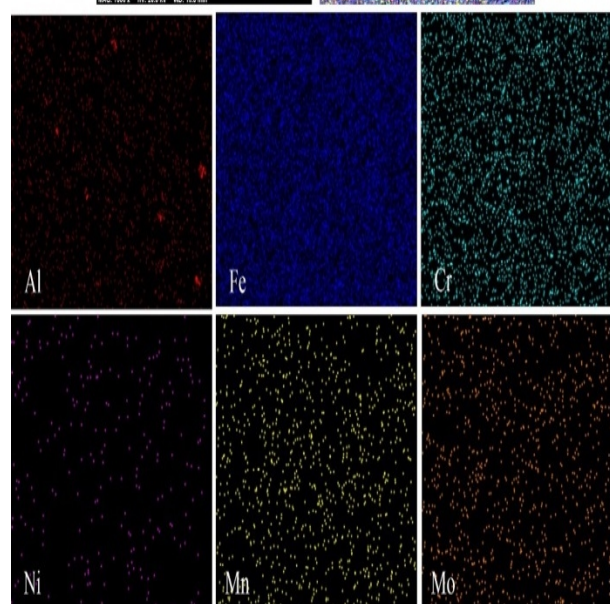
شکل 11- آنالیز نقشه عنصری EDS ناحیه مرکزی لایه روکش (Fe, Cr)_3Al
