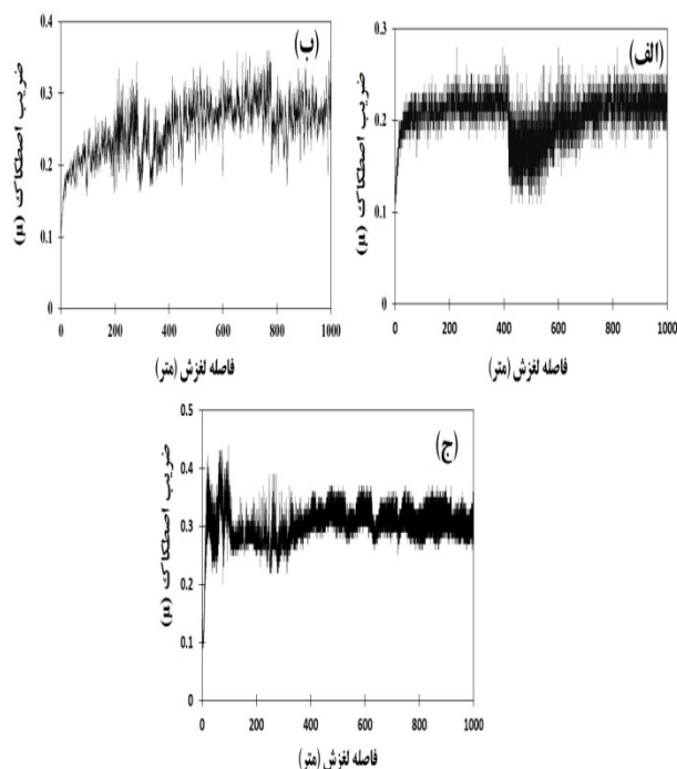
شکل 16- ضریب اصطکاک برحسب مسافت لغزش برای پین‌های پوشش داده شده توسط Fe_3Al در دماهای (الف) 25 درجه سانتی‌گراد، (ب) 200 درجه سانتی‌گراد و (ج) 500 درجه سانتی‌گراد
