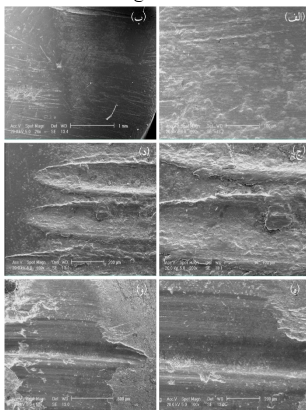
شکل 18- تصاویر SEM از سطح سایش روکش (\text{Fe,Cr})_3\text{Al} در دماهای،
