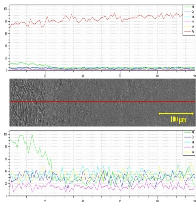
شکل 6- آنالیز عنصری خطی EDS از ناحیه پوشش \text{Fe}_3\text{Al} تا منطقه متأثر از حرارت
