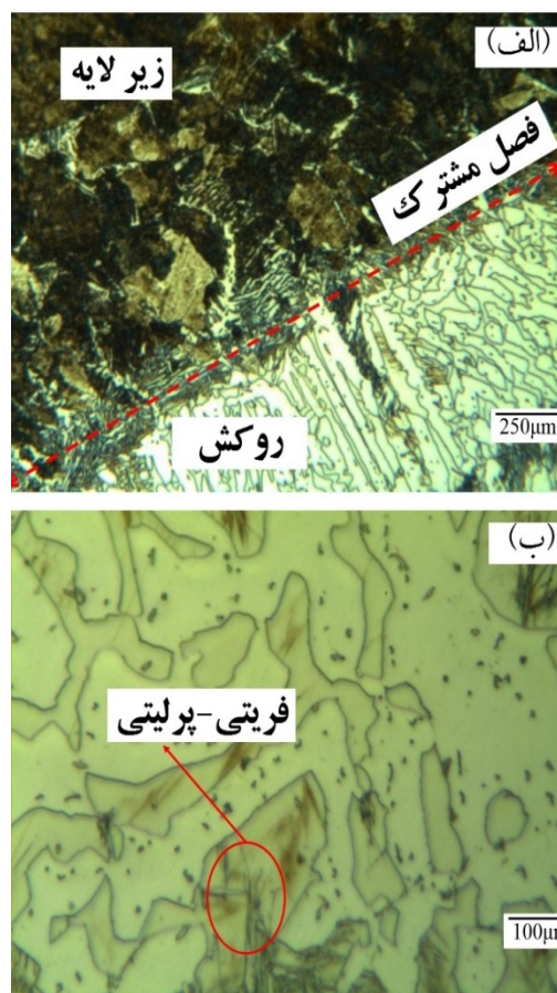
شکل 4- ریزساختار سطح مقطع پوشش \text{Fe}_3\text{Al} ، (الف) ریزساختار فصل مشترک پوشش/زیرلایه و (ب) ریزساختار پوشش \text{Fe}_3\text{Al} .
