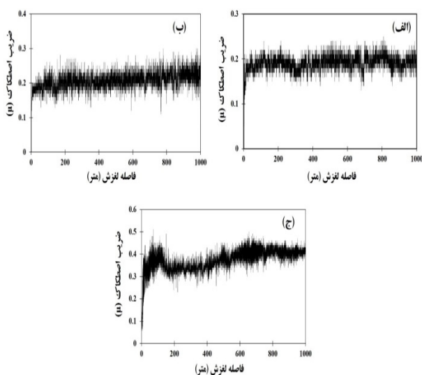
شکل 20- نمودار تغییرات ضریب اصطکاک بر حسب مسافت لغزش برای روکش (Fe, Cr)_3Al در دماهای الف - 25 °C، ب - 200 °C و ج - 500 °C
