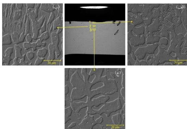
شکل 5- تصاویر SEM از پوشش \text{Fe}_3\text{Al} : الف - ناحیه بالایی (نقطه 1)، ب - ناحیه میانی (نقطه 2) و ج - منطقه پایینی روکش (نقطه 3).
