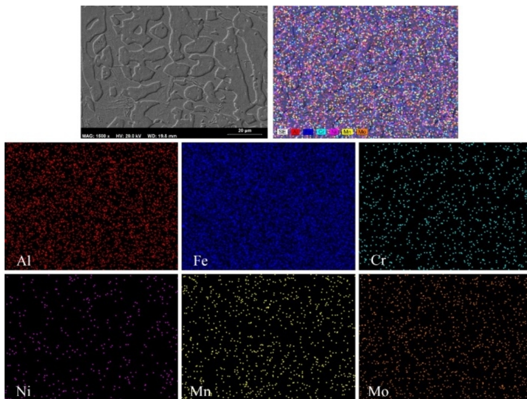
شکل 7- آنالیز نقشه عنصری EDS مرکز پوشش \text{Fe}_3\text{Al}
