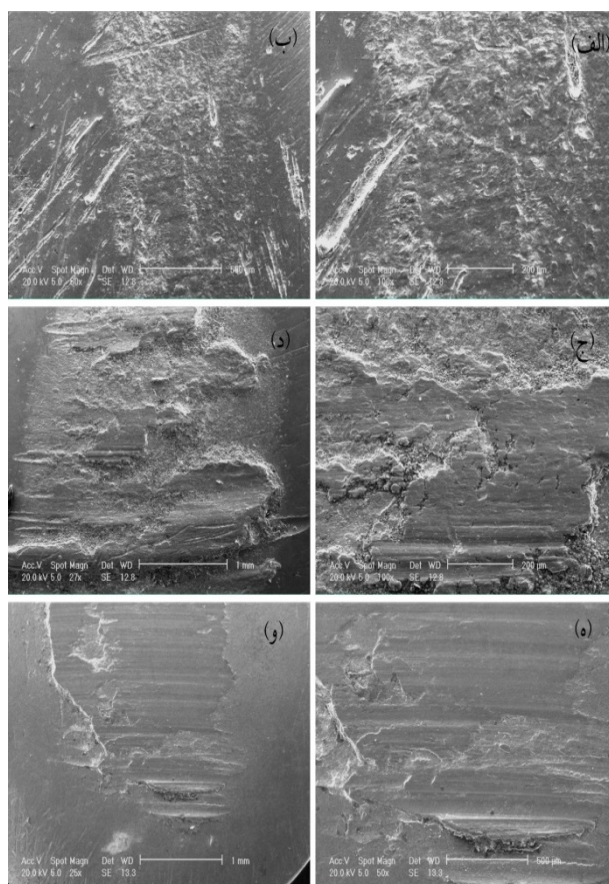
شکل 14- تصاویر SEM از سطح سایش پین روکش Fe_3Al در دماهای، (الف و ب) 25°C، (ج و د) 200°C و (و و ه) 500°C.
