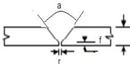
شکل 1- شماتیک طرح اتصال جوشکاری شده.
