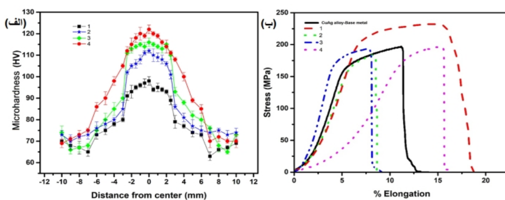
شکل 8-الف - نمودار ریزسختی سنجی ویکرز نمونه FSP شده بدون ذرات تقویت کننده (نمونه 1)، کامپوزیت Cu-Ag-SiC با ذرات تقویت کننده میکرو در مقادیر مختلف 0/02 گرم (نمونه 2) و 0/04 گرم (نمونه 3) و کامپوزیت Cu-Ag-SiC با ذرات تقویت کننده نانو (نمونه 4) و ب- منحنی‌های تنش-ازدیاد طول نمونه‌های خام، 1، 2، 3 و 4-تأثیر فرایند FSP و اندازه ذرات و مقدار تقویت کننده SiC نانومتری و میکرومتری.
