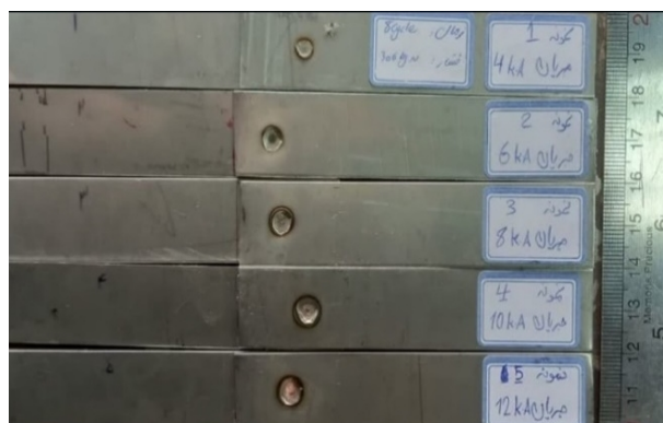
شکل 3- نمونه‌های جوشکاری شده بدون لایه واسط.
