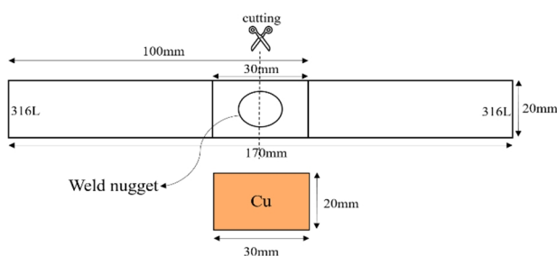
شکل 1- طرح‌واره و ابعاد نمونه‌های جوشکاری شده.
