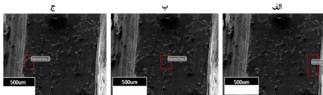
شکل 10- نتایج آزمون طیفسنجی پراکندگی انرژی پرتو ایکس به صورت زمینه ای مربوط به نمونه با لایه واسط.
