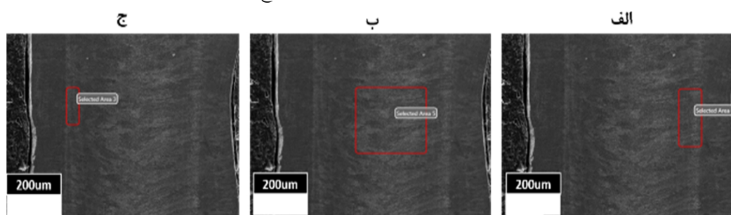
شکل 11- نتایج آزمون طیفسنجی پراکندگی انرژی پرتو ایکس به صورت زمینه ای مربوط به نمونه بدون لایه واسط.
