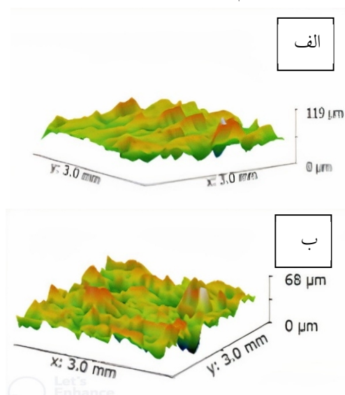
شکل 4- پروفیل زبری نمونه‌های 120-980 بعد از الف- برشکاری و ب- سنباده‌زنی و پولیش کاری.
