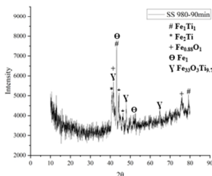
شکل 8-آنالیز پراش پرتو ایکس از سطح نمونه شکست 980-90.
