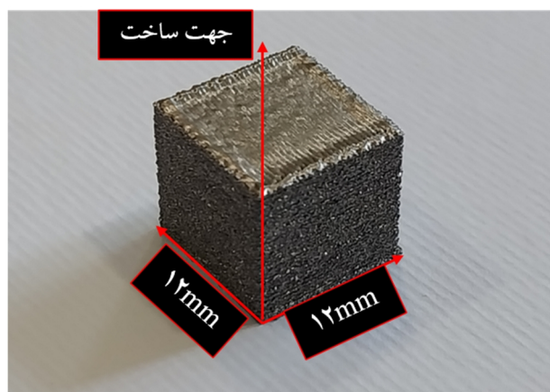
شکل 1- تصویر قطعات مکعبی آلیاژ Ti-6242 (EBM).
