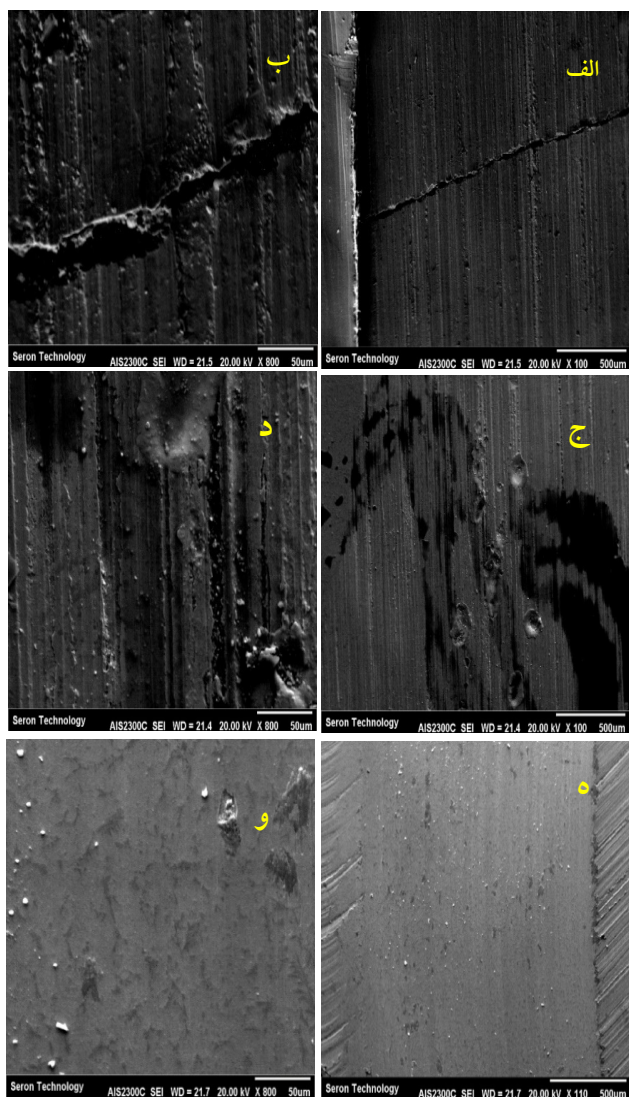
شکل 11- تصاویر شیار سایش روکش کلمونوی به روش قوس پلازما بعد از سایش در دمای محیط (الف و ب)، بعد از سایش در دمای 300 درجه (ج و د) و بعد از سایش در دمای 600 درجه (ه و و)
