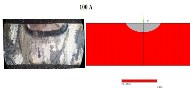
شکل 9- مقایسه شکل حوضچه جوش به دست آمده از آزمایش های مدل عددی (سمت راست) و عملی (سمت چپ).
