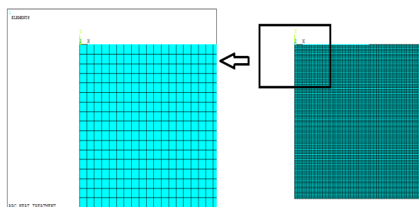
شکل 1- مش‌بندی مورد استفاده در شبیه‌سازی المان محدود.
