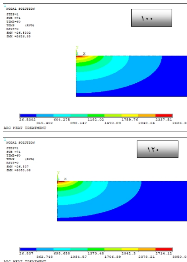
شکل 8- توزیع دما در نمونه های با شدت جریان الف - 100 و ب - 120 آمپر.
