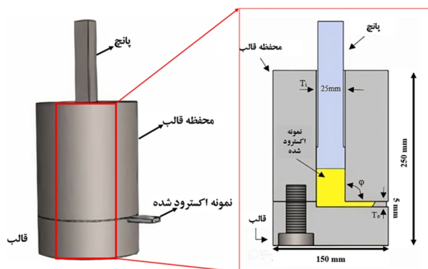
شکل 1- طرحواره قالب اکستروژن تجمعی زاویه ای [10].
