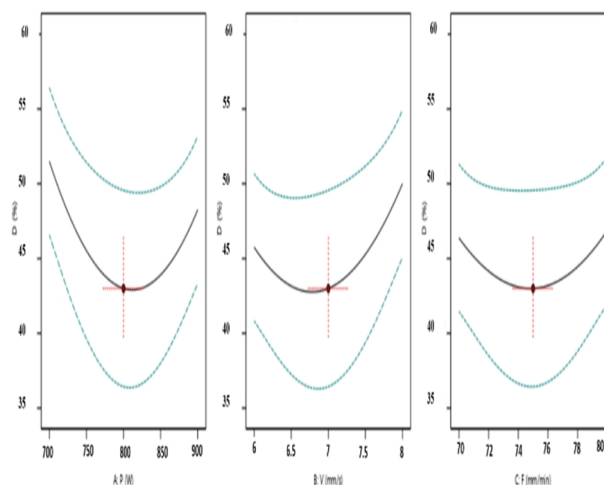
شکل 13- رابطه پارامترهای اصلی با میزان آمیختگی تک‌پاس.
