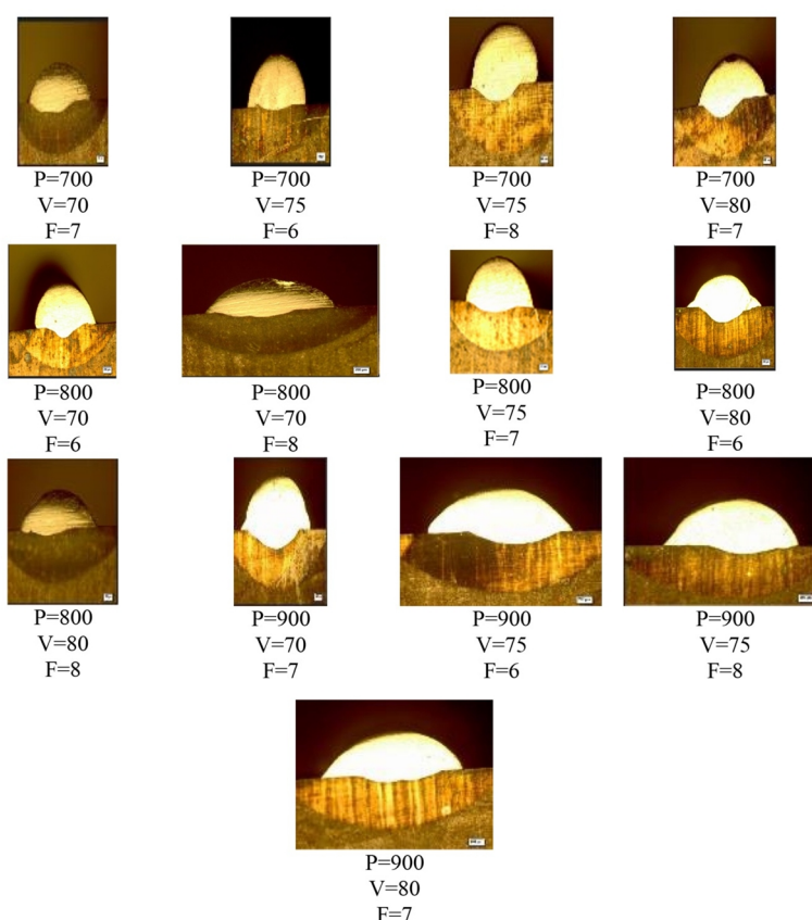
شکل 5- تصاویر میکروسکوپ نوری از مقطع نمونه های تک پاس
