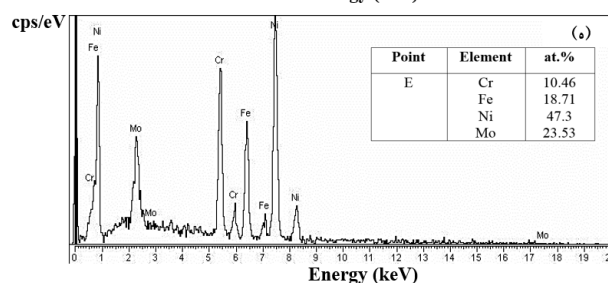
شکل 7- نتایج آنالیز عنصری فازهای الف - تیغه‌ای، ب - دندردیتی، ج - فصل مشترک، د - کروی و ه - زمینه.
