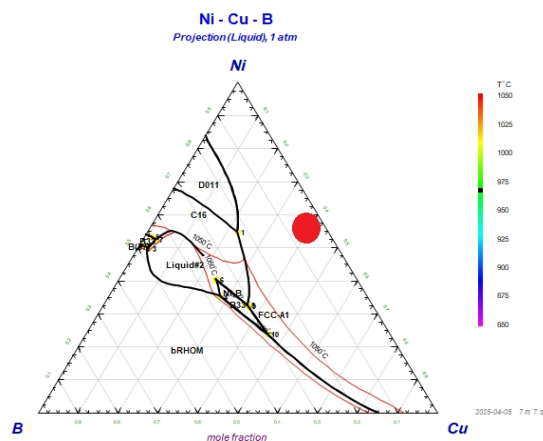
شکل 3- نمودار سه‌تایی نیکل - مس - بور.
