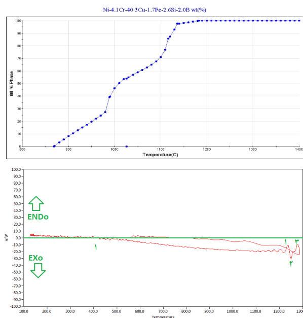
شکل 4- نمودار حرارتی
