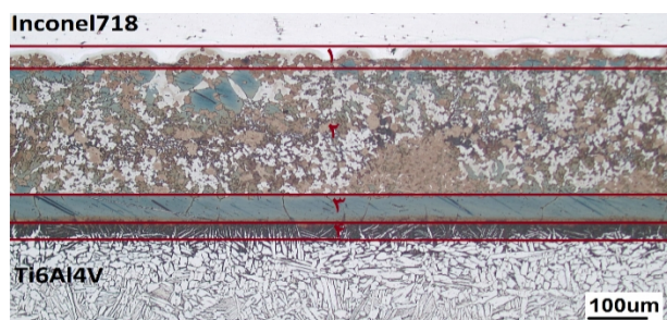
شکل 6- تصویر متالوگرافی از مناطق مختلف اتصال بهینه در دما و زمان 950°C - 20 دقیقه.
