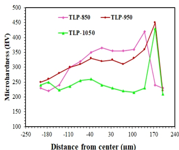
شکل 13- پروفیل میکروسختی از سطح مقطع نمونه های اتصال.
