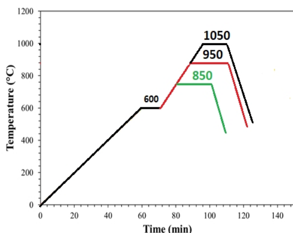
شکل 2- گراف دما - زمان فرایند اتصال‌دهی Ti-6Al-4V به اینکونل 718.
