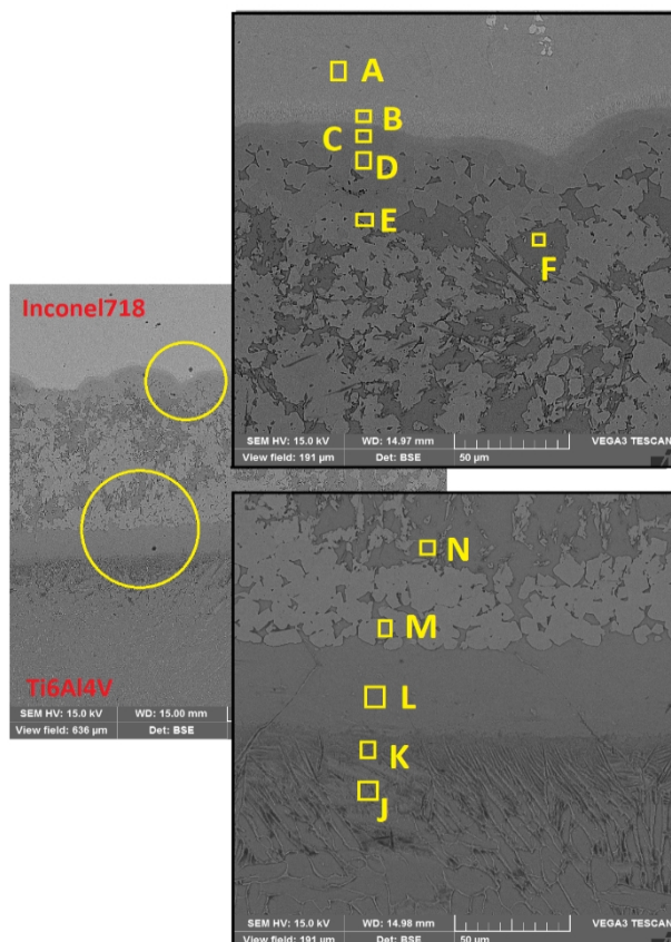
شکل 7- تصویر میکروسکوپ SEM نمونه اتصال داده شده در دمای 950^{\circ}\text{C} و زمان 20 دقیقه.
