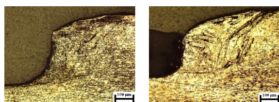
شکل 7- تصویر ماکروسکوپی کنار جوش نمونه با مدت زمان تماس 40 ثانیه و سرعت دورانی 1320 (الف)، 1800 (ب) و 2500 (پ)
