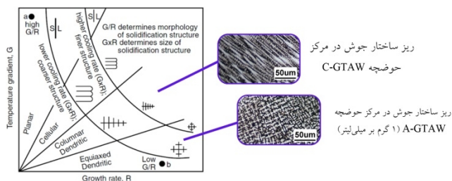
شکل 18. نمودار اثر گرادیان دمایی و نرخ رشد بر مورفولوژی‌های انجمادی ممکن در منطقه مذاب جوش نشان می‌دهد [4]. ریزساختارهای نشان داده شده مربوط به تصاویر OM پژوهش حاضر است که از منطقه مشابه تهیه شده است.
