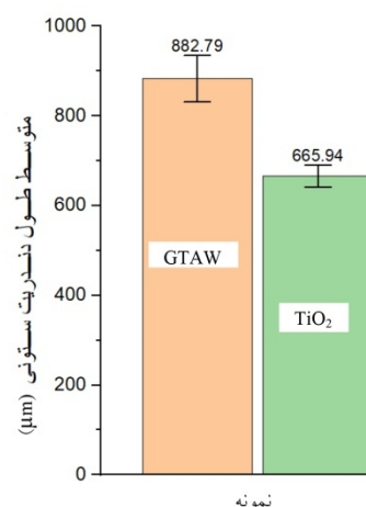
شکل 19-مقایسه طول دندریته های ستونی نمونه ها با یکدیگر.
