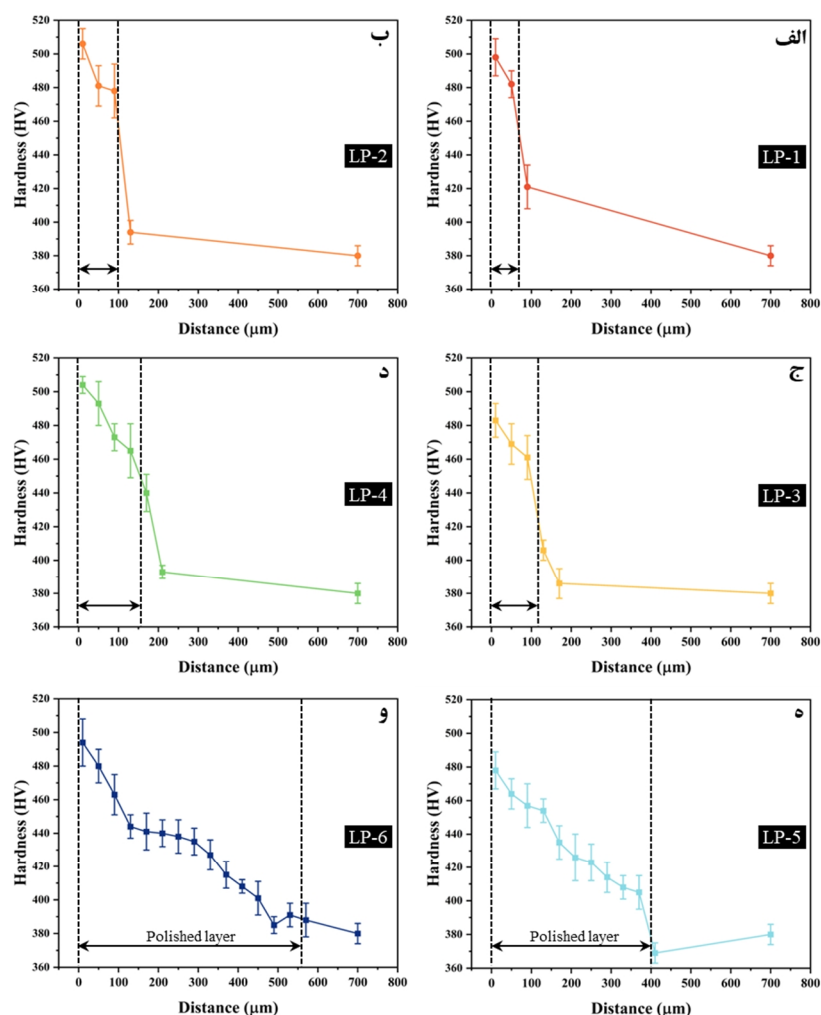
شکل 8- تغییرات مقادیر سختی نمونه‌های الف- LP-1، ب- LP-2، ج- LP-3، د- LP-4، هـ- LP-5 و و- LP-6 با فاصله گرفتن از سطح قطعه (پیکان ضخامت لایه پولیش شده را نشان می‌دهد).
