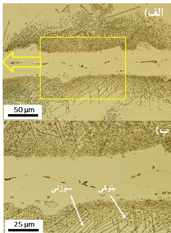
شکل 3- رسوبات شکل گرفته در DAZ الف- نمونه °C 1150- 5s و °C 1120- 24min، ب- الف در بزرگنمایی بیشتر.
