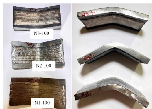
شکل 10- نمونه‌های یک پاس، دو پاس و سه پاس روکش‌کاری شده با دمای پیشگرم 100°C پس از انجام آزمایش خمش.
