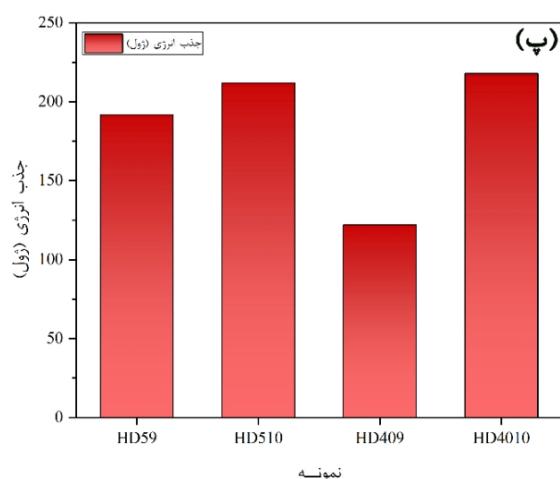
شکل 3- نتایج حاصل منحنی نیرو- جابجایی در دو جریان 9 و 10 کیلوآمپر و زمان نگهداری 5 و 40 سیکل، الف- حداکثر نیرو، ب- جابجایی و پ- میزان انرژی جذب شده برای شکست.
