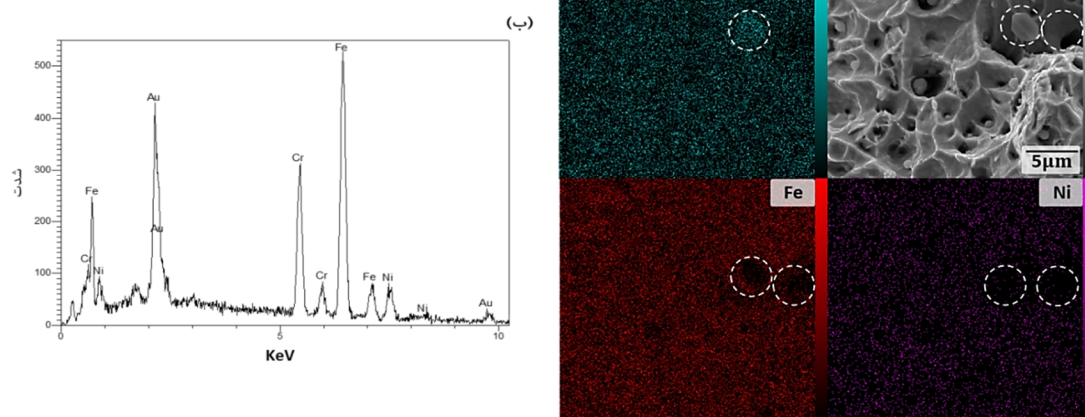
شکل 9- الف - نقشه توزیع غلظت عناصر Cr، Ni، Au و Fe و ب - پیک حاصل از آنالیز نقطه ای EDS در مقطع شکست نمونه الف آزمون کشش.
