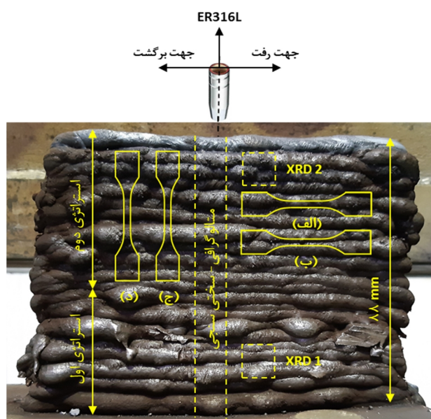
شکل 2- دیوار نازک SS316L ساخته شده به روش WAAM و تعیین محل استخراج نمونه‌های مورد آنالیز ریزسختی، فازی و آزمون‌های خواص مکانیکی.
