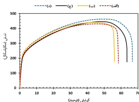
شکل 7- نمودارهای حاصل از آزمون کشش دیوار نازک SS316L ساخته شده: الف و ب- نمونه های افقی و (ج و د) عمودی.
