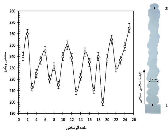
شکل 10- نمودار سختی کل دیوار نازک ساخته شده SS316L به روش WAAM با تعیین موقعیت‌های اثر سختی.
