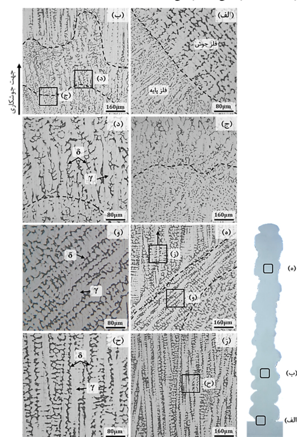
شکل 5- تصاویر ریزساختاری از بخش‌های مختلف دیوار نازک SS316L ساخته شده به روش WAAM.
