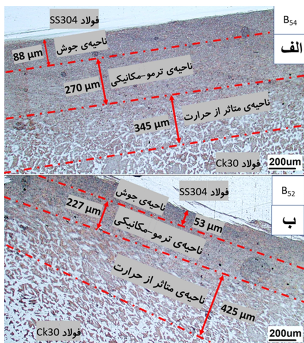
شکل 10- تصویر میکروسکوپ نوری از ریزساختار کلی منطقه جوش دو نمونه الف - B 54 و ب - B 52 در سمت ساده کربنی.
