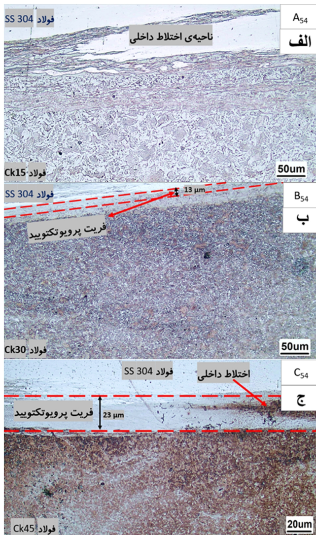
شکل 8- تصاویر میکروسکوپ نوری از ریزساختار ناحیه جوش سه نمونه الف - A_{54} ، ب - B_{54} و ج - C_{54} در سمت ساده کربنی.
