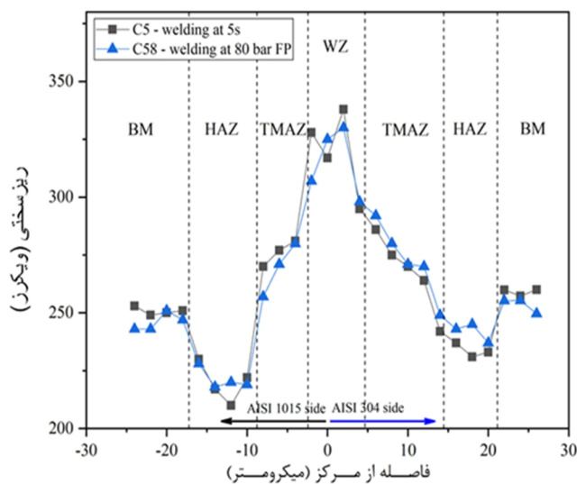
شکل 15- نتایج آزمایش ریزسختی بر روی نمونه‌های سری C.
