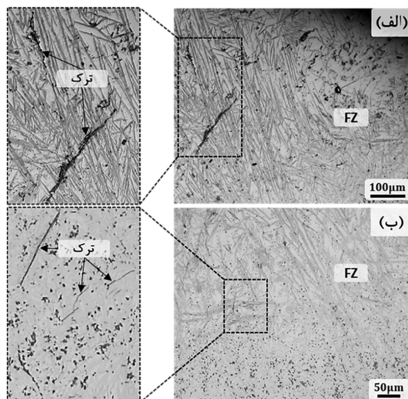
شکل 9- تصویر میکروسکوپی نوری از ترک‌های موجود در بخش فلز جوش چدن خاکستری جوشکاری شده به روش SMAW با الکترود E6013.
