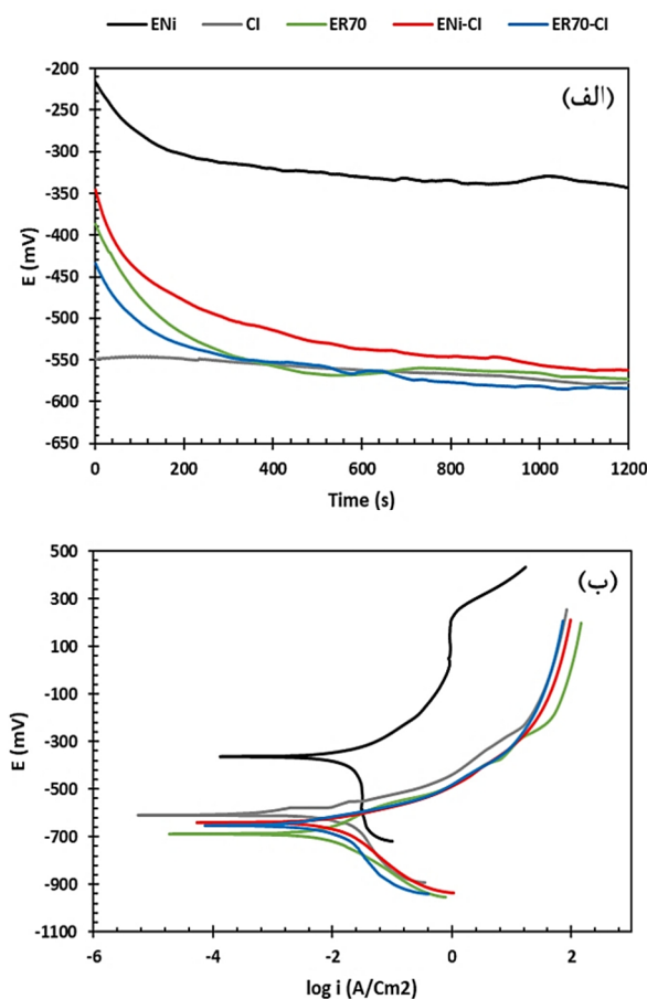
شکل 14- منحنی آزمون‌های خوردگی نمونه‌های غوطه‌ور در محلول 3/5 درصد NaCl: الف - OCP و ب - PDP.
