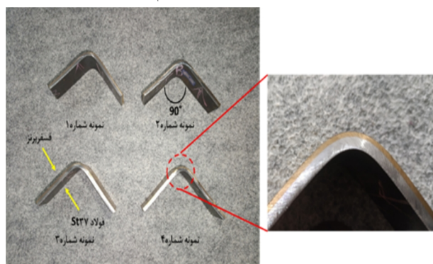
شکل 14- مورفولوژی ماکروسکوپی نمونه های جوشکاری شده پس از 90 درجه خم شدن
