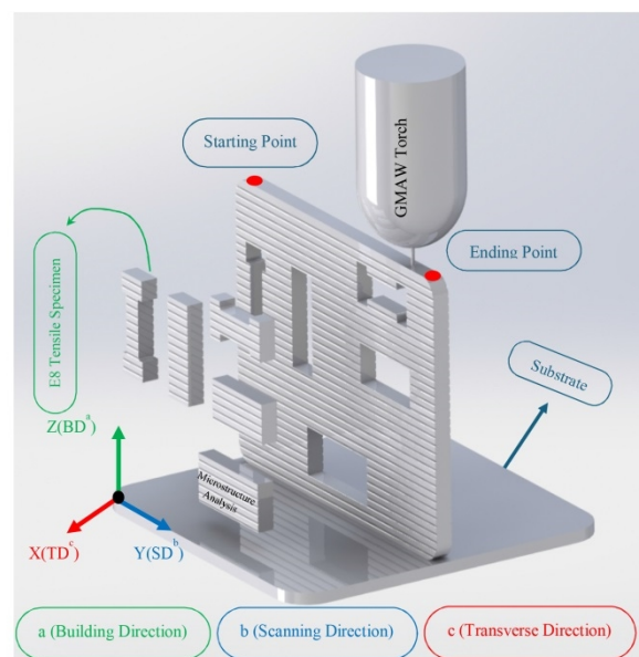
شکل 2- طرحواره دیواره فولاد زنگ‌نزن L316 ساخته شده توسط فرایند ساخت افزایشی قوسی سیمی همراه با نمونه‌های آزمایش کشش و آنالیز ریزساختاری.
