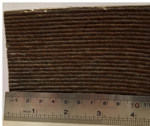
شکل 1- دیواره فولاد زنگ نزن 316 ساخته شده با فرایند ساخت افزایشی قوسی سیمی.
