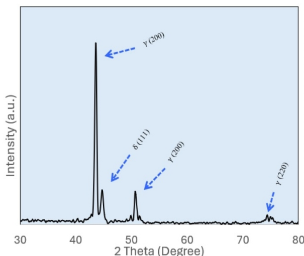
شکل 7- الگوی پراش اشعه ایکس (XRD) فولاد زنگ‌نزن آستنیتی 316L تولید شده با فرایند WAAM
