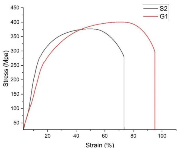
شکل 21- نمودار تنش- کرنش نمونه‌های آزمون کشش: S2، GMAW - G1 - SMAW
