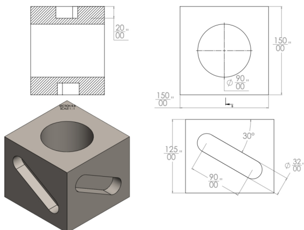
شکل 9- نمایش بصری و شبیه سازی شده جزئیات هندسی اتصال شفت به پره، با ابعاد بر حسب میلی متر.
